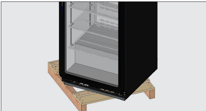
Abb. 4. Drehen Sie das Gerät auf der Kufe. Verwenden Sie beim Hochheben des Geräts keine Arbeitsplatten, Türen/Schubladen oder Gitter als Hebepunkte.
