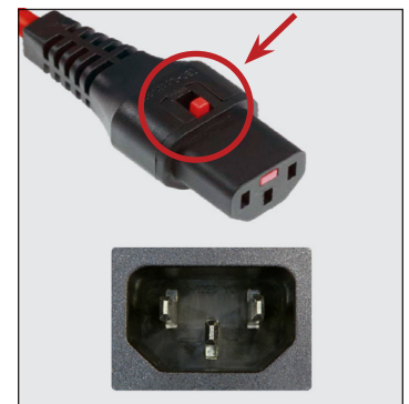
Rys. 2. Nacisnąć czerwony przycisk, aby wyjąć wtyk.
